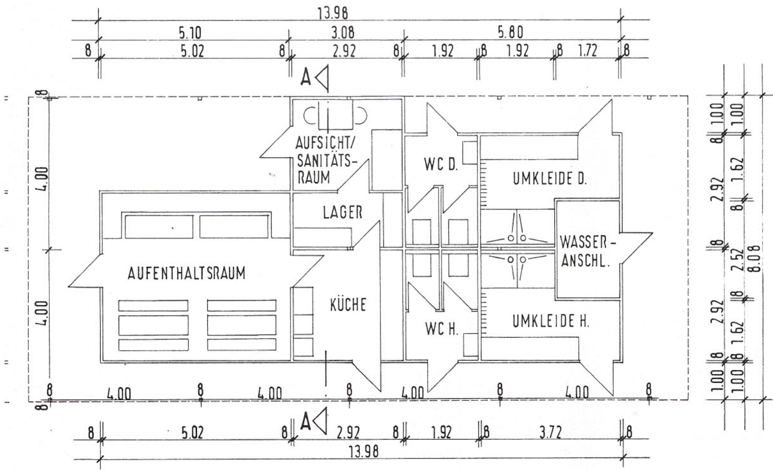
GRUNDRISS EG.
